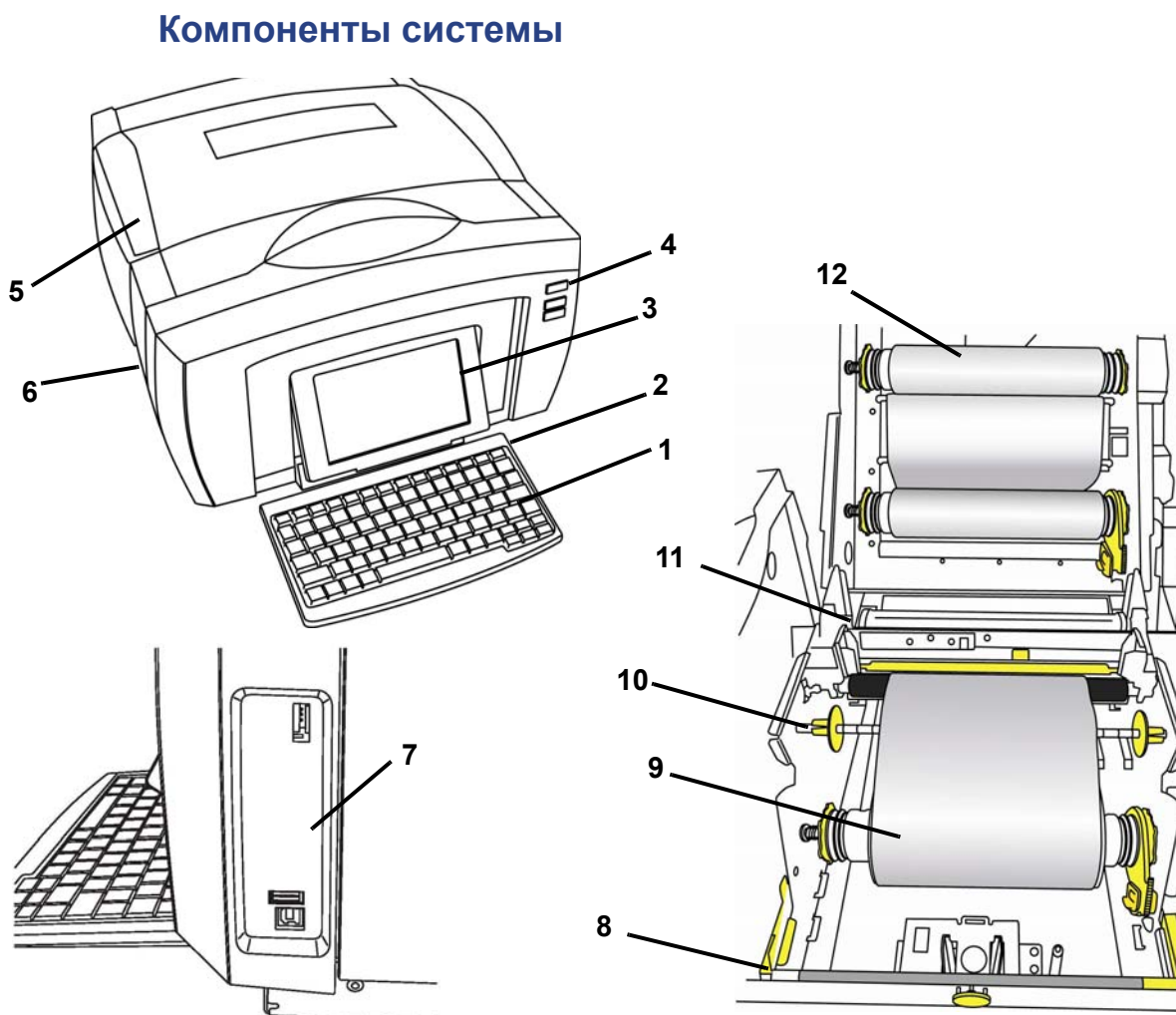
Рис. 2-1. Компоненты принтера
